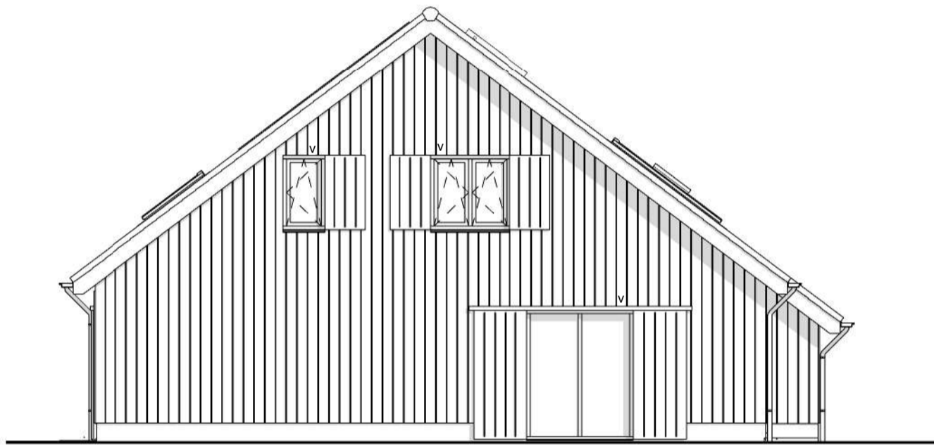
Kavel 12 en 14 Rechterzijgevel
