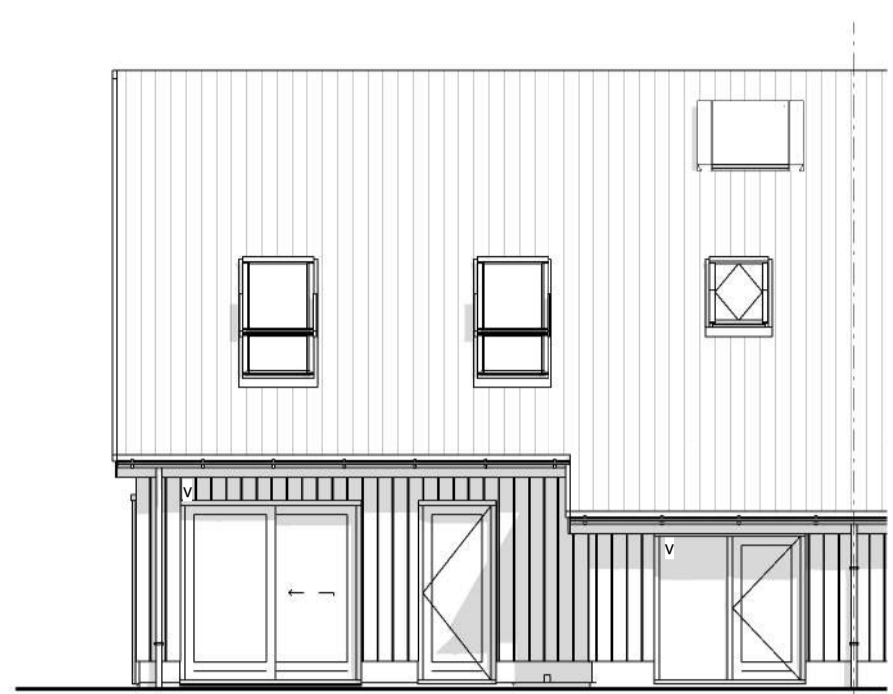
Kavel 12 en 14 Achtergevel
