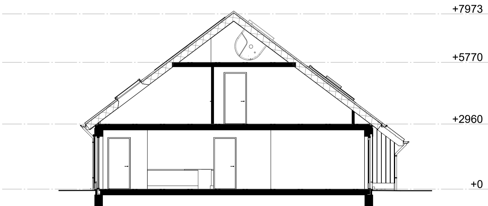
Kavel 12 en 14 doorsnede
