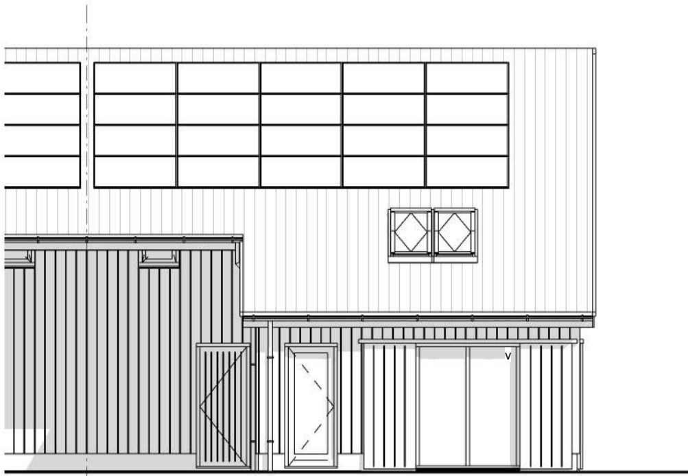
Kavel 12 en 14 Voorgevel
