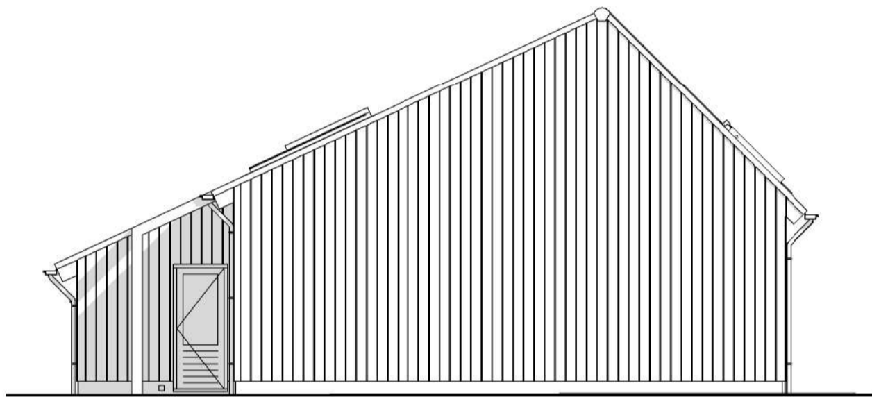
Kavel 3 linkerzijgevel
