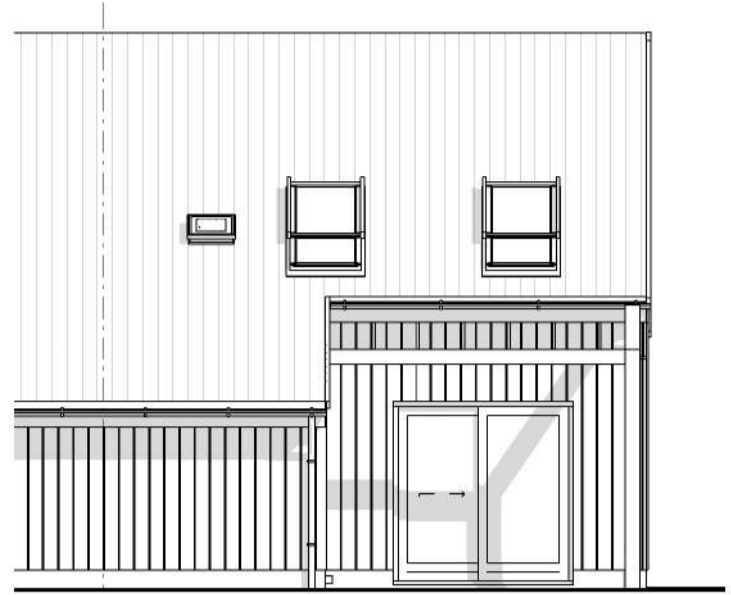
Kavel 3 Achtergevel
