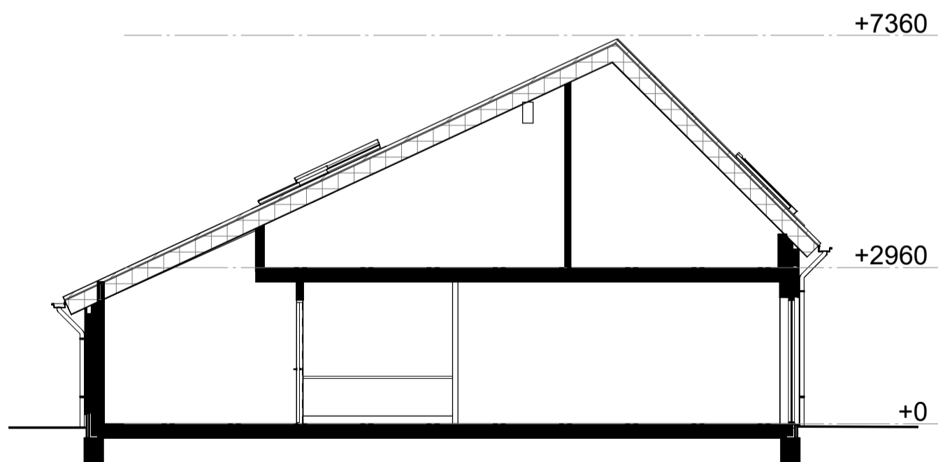
Kavel 3 doorsnede
