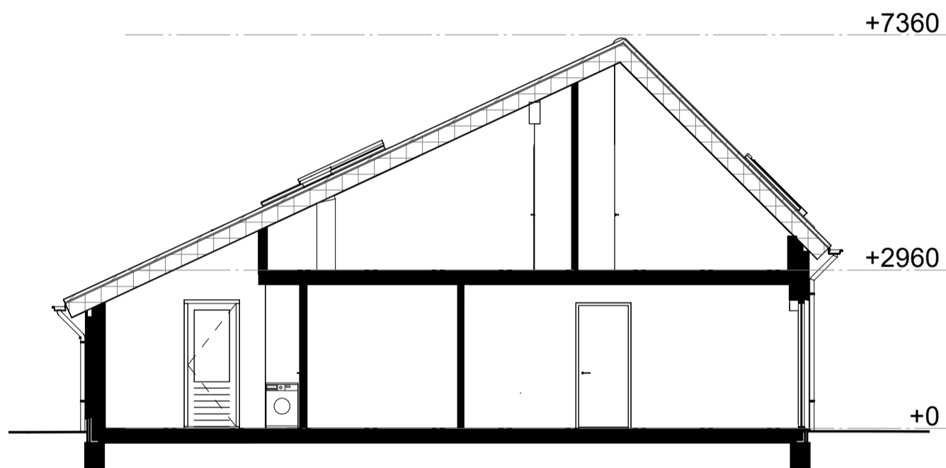
Kavel 4 en 8 Linkerzijgevel
