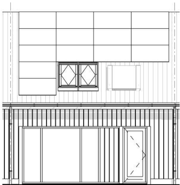
Kavel 4 en 8 Voorgevel
