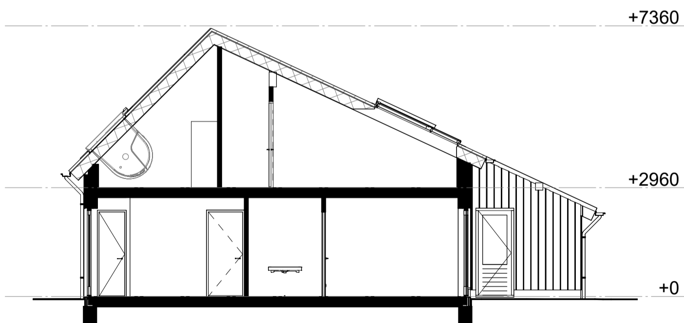
Kavel 4 en 8 Doorsnede
